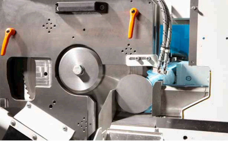
Sägeblatt mit Führung und Spannung.
